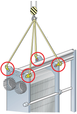
그림 5: T45, TL35 및 WideGap 350용 인양 장치. 고정 장비가 필요하지 않습니다.
