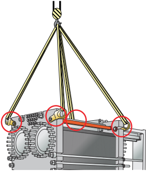
그림 6: T50용 인양 장치. 고정 장비가 필요합니다.
