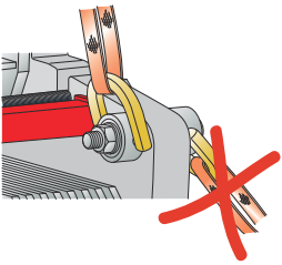
그림 7: TS50용 인양 장치. 열교환기 인양 시 내부 아이 볼트 4개를 사용하십시오. 운송 고정 포인트를 사용하지 않아야 합니다. 고정 장비가 필요합니다.
