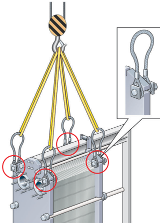
그림 4: T35 및 TS35용 인양 장치. 고정 장비가 필요합니다.
