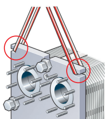
Figura 4: Ridicare M3, M6, M10, T2, T5, TS6, TL3 și versiunea veche a T8, TL6
