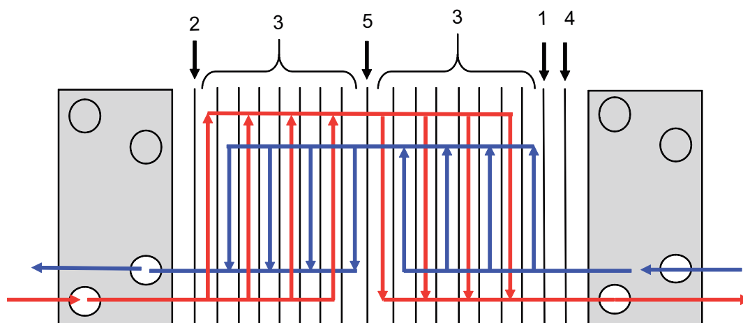
Figura 3: Exemplu de configurație cu mai multe treceri.
