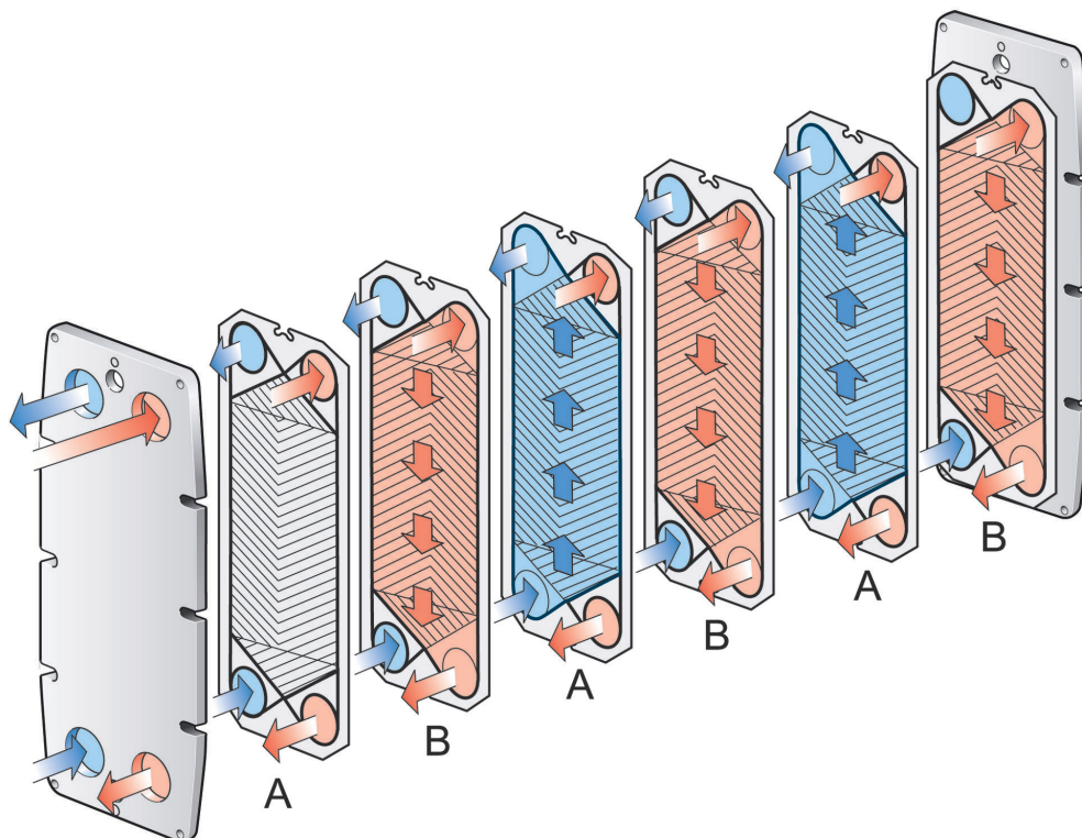
Рис. 2: Схема расположения набора пластин, прокладки обращены к опорной пластине.
