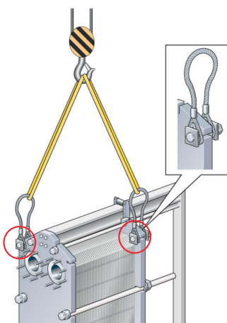
Figura 4: Dispozitiv de ridicare pentru AQ6, AQ4L, AQ6L, AQ8 și AQ8S.
