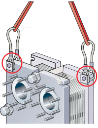
图 7: 起吊 T10、(T6)、T8、TL6
