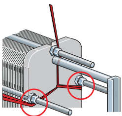
图 6：起吊 TS6。
