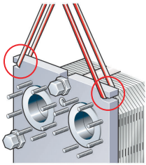
图 4：起吊 M3、M6、M10、T2、T5、TS6、TL3 以及旧版 T8、TL6
