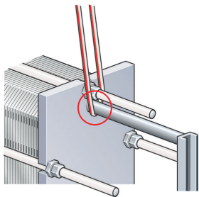
图 5：起吊 M3、M6、M10、T2、T5、TL3 以及旧版 T8、TL6
