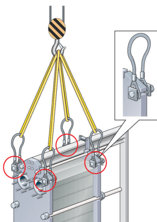
Figure 6 : Dispositif de levage pour les modèles T25, MX25 et MA30-S.
