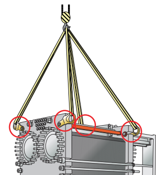
Kuva 7: Nostolaite mallille T50. Kiinnitysvälineitä on käytettävä.
