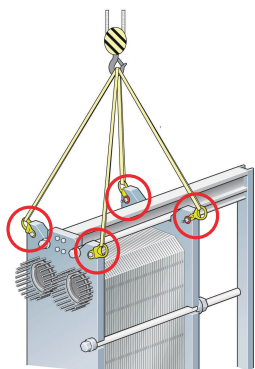
Kuva 6: Nostolaite malleille T45, TL35 ja WideGap 350. Kiinnitysvälineitä ei vaadita.
