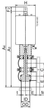
Valvola deviatrice
