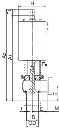
Valvola di intercettazione
