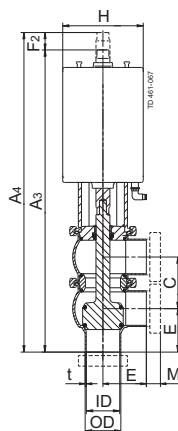
Valvola deviatrice
