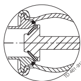
PTFE プラグ・シール (TR2)
