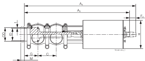
切り替えバルブ
