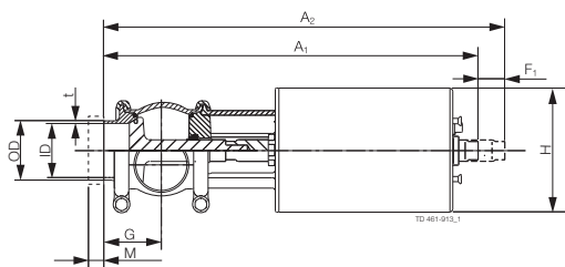
開閉バルブ
