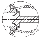
Tenuta otturatore PTFE (TR2)
