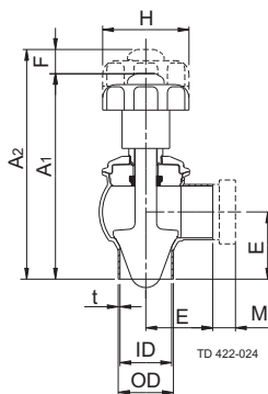
図 4. 寸法
