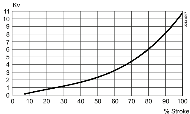
Fig. 3. La portata in % rispetto alla portata totale con una perdita di carico di 1 bar.
