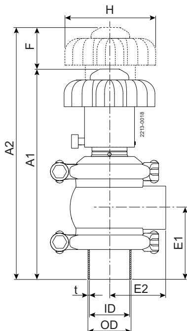
Obr. 4. Rozměry
