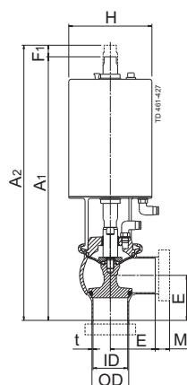
開閉バルブ
