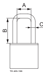
Obr. 2. Rozměry - visací zámek. Obr. 3. Polohový kryt. A. Min. 20 mm B. Min. 35 mm C. \varnothing 6 mm 1. Zap/vyp 2. Vícepolohové
