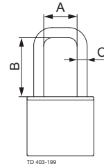
图 2. 尺寸 - 挂锁 A. 最低 20 mm B. 最低 35 mm C. \varnothing 6\text{ mm}
