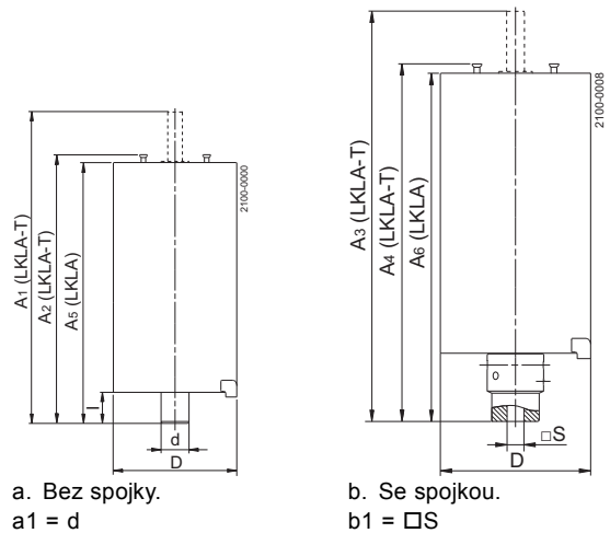
Obr. 2. Rozměry - pohon
