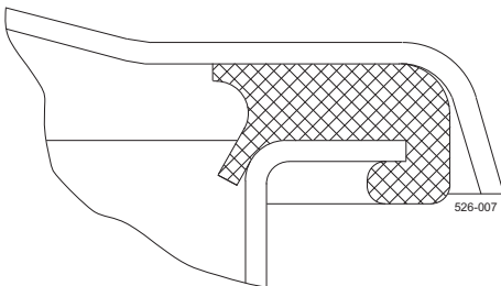
Kuva. 2. Kaksitoiminen huultiviste
