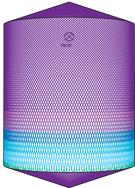
D5m H6m, Toftejorg TZ-74 versione autopulente, 4 x \varnothing 7 mm, 0% tempo = 15.3 min., consumo acqua = 4853 l
