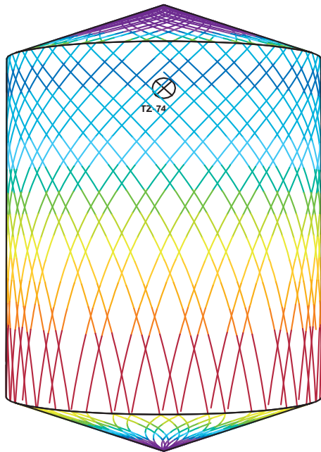
D5m H6m, Toftejorg TZ-74 versione autopulente, 4 x \varnothing 7 mm, 0% tempo = 3.8 min., consumo acqua = 1192 l
