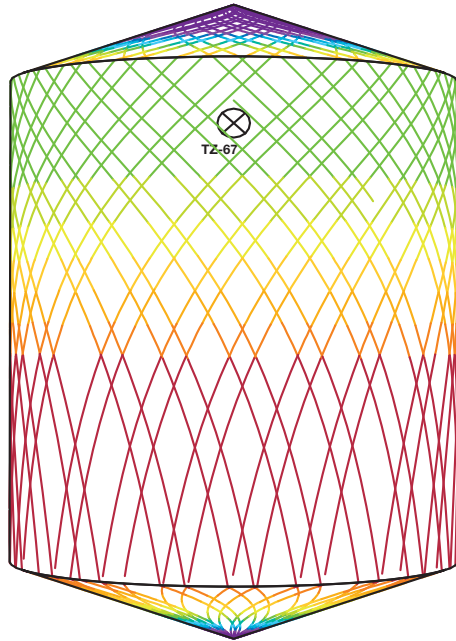
D2,5 m H6m, Toftejorg TZ-67, 4 x \varnothing 6 mm Tempo = 35 min., consumo acqua = 727 l
