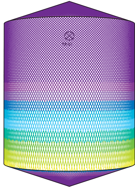
D2,5 m H6m, Toftejorg TZ-67, 4 x \varnothing 6 mm Tempo = 147 min., consumo acqua = 3097 l
