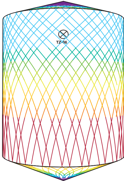
D8m H10m, Toftejorg TZ- 66, 4 x ø10 mm, 0% Tempo = 5.5 min., consumo acqua = 2565 l
