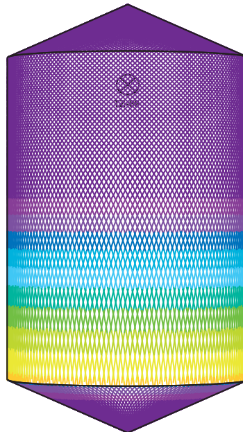
D2m H3m, Toftejorg TZ-89, 4 x φ4 mm Aika = 11.1 min, vedenkulutus = 637 l
