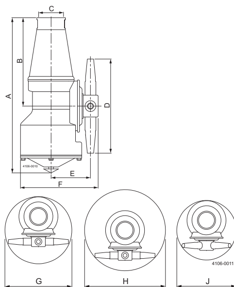
寸法 (mm)
