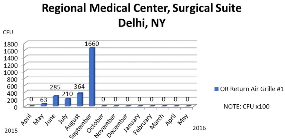
Chart 'B3': OR Return Air Grille #1
